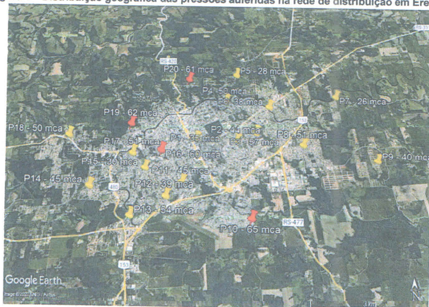
Figura 1 – Distribuição geográfica das pressões auferidas na rede de distribuição em Erechim
